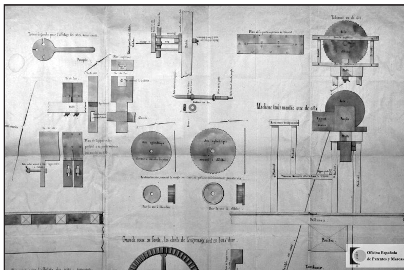
Màquina de fabricació de pipes de bruc per a la qual Francesc Xavier Fonalleras va demanar un privilegi d'introducció el 14 de maig de 1860. Font: Sáiz, P.; Llorens, F.; Blázquez, L.; y Cayón, F. (Drs.): Base de datos de solicitudes de patentes (España, 1878-1939), OEPM-UAM, Madrid, 2000-2008, http://historico.oepm.es
